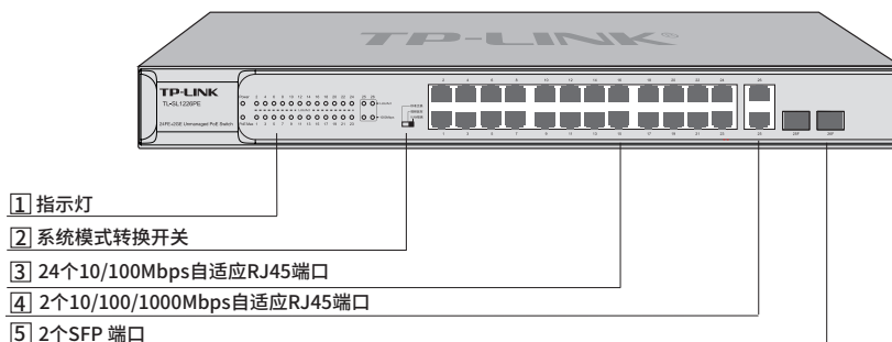
图1-6 TL-SL1226PE前面板示意图
