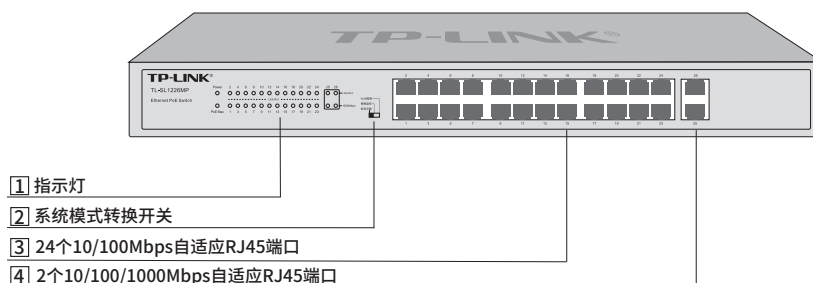
图1-2 TL-SL1226MP前面板示意图
