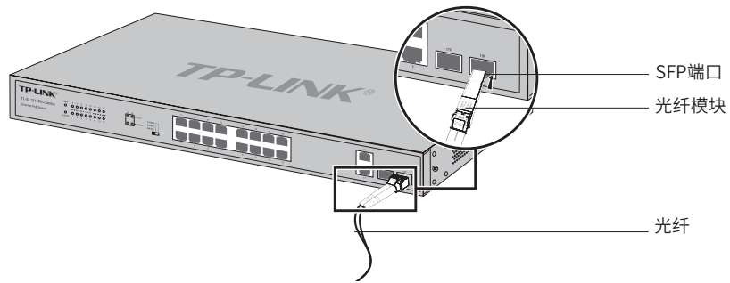
图3-2 SFP端口连接示意图
