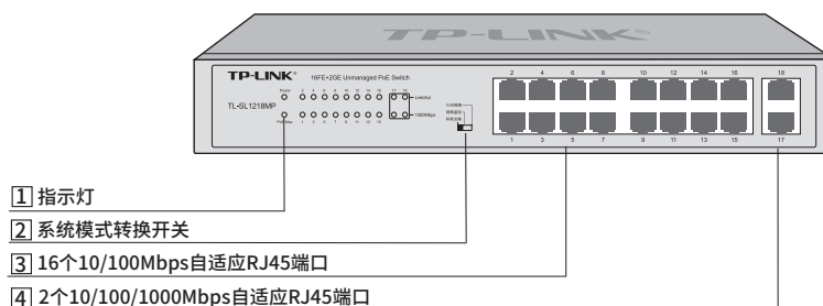
图1-1 TL-SL1218MP前面板示意图
