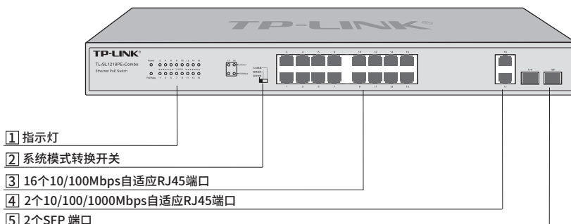
图1-5 TL-SL1218PE-Combo前面板示意图
