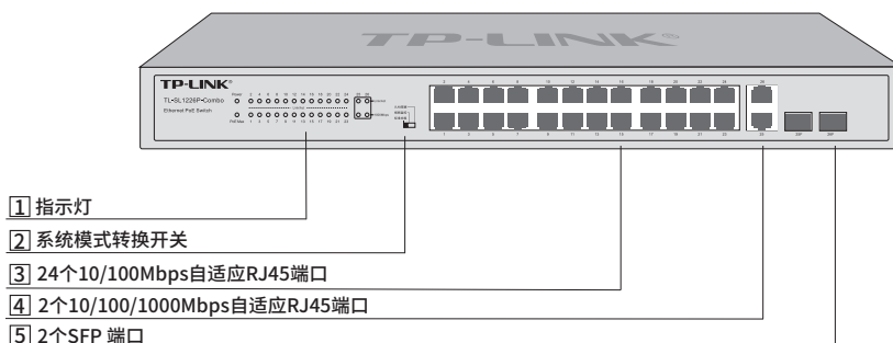
图1-4 TL-SL1226P-Combo前面板示意图
